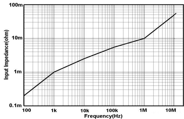
图 6 HCP8150G 输入阻抗 VS 频率曲线
