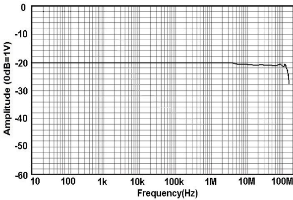
图 1 HCP8030G 幅频曲线
