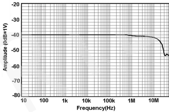
图 4 HCP8150G 幅频曲线
