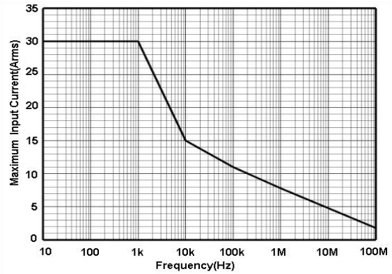
图 2 HCP8030G 最大测量电流 VS 频率曲线 (超过该曲线所示最大电流连续使用会导致探头烧毁)
