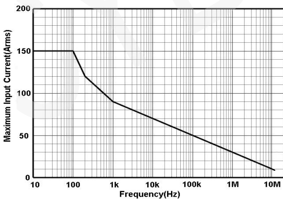
图 5 HCP8150G 最大测量电流 VS 频率曲线 (超过该曲线所示最大电流连续使用会导致探头烧毁)
