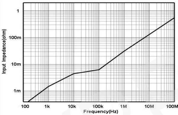
图 3 HCP8030G 输入阻抗 VS 频率曲线
